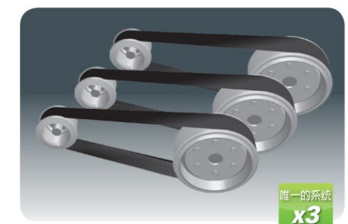
1套传送皮带 2套标准皮带轮
