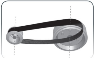
不使用工具在大皮带轮上安装并调整传动皮带
