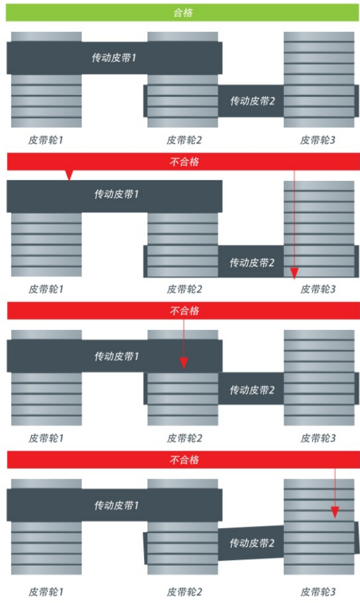
使用SNAP ON工具在大皮带轮上安装并调整传动皮带
