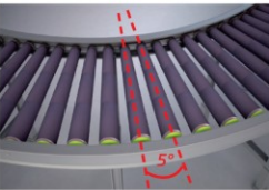
该配置在转弯式输送机上同样有效。
